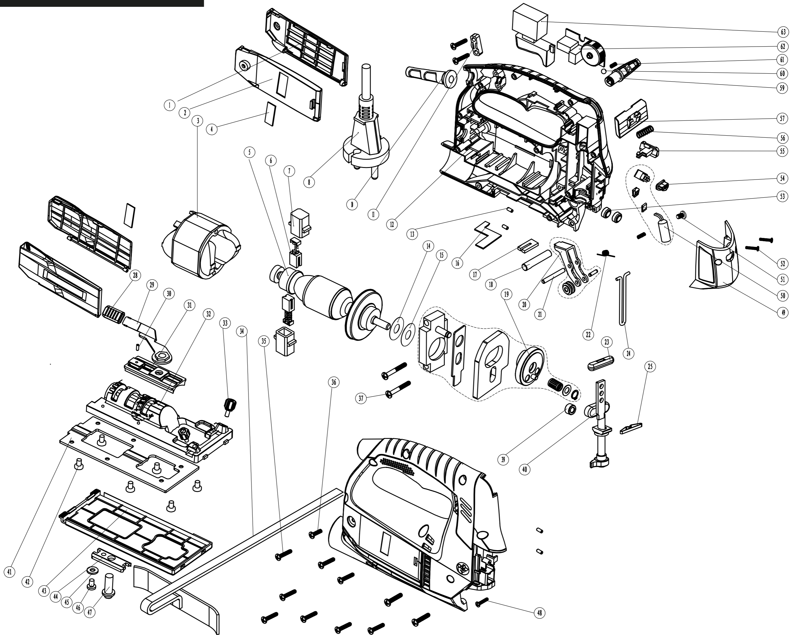
51.01-PRP-800 | pila přímočará 800W
